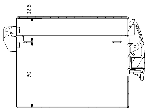
COUPE A-A
