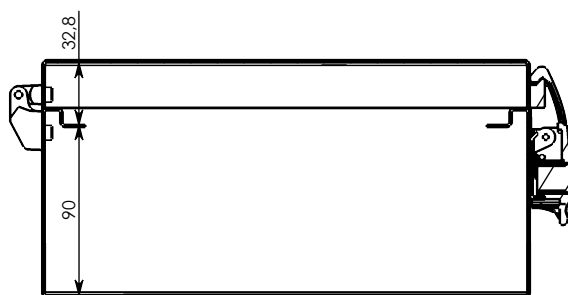
COUPE A-A
