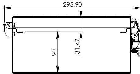
COUPE A-A
